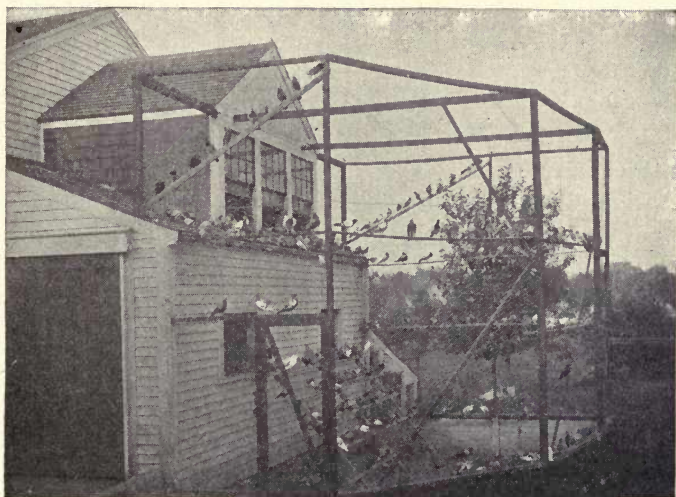
FIG. 87—A Pigeon Loft.
